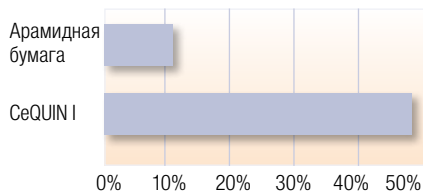
Поглощение влаги
