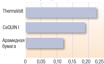
Впитывание лака
