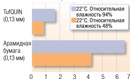
Поглощение влаги
