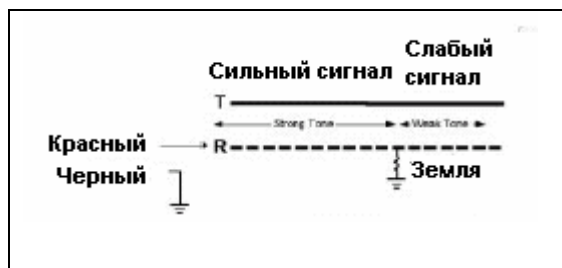
Рисунок 3. Подключите зажим красного цвета к поврежденному проводнику, зажим черного цвета к заземлению.
